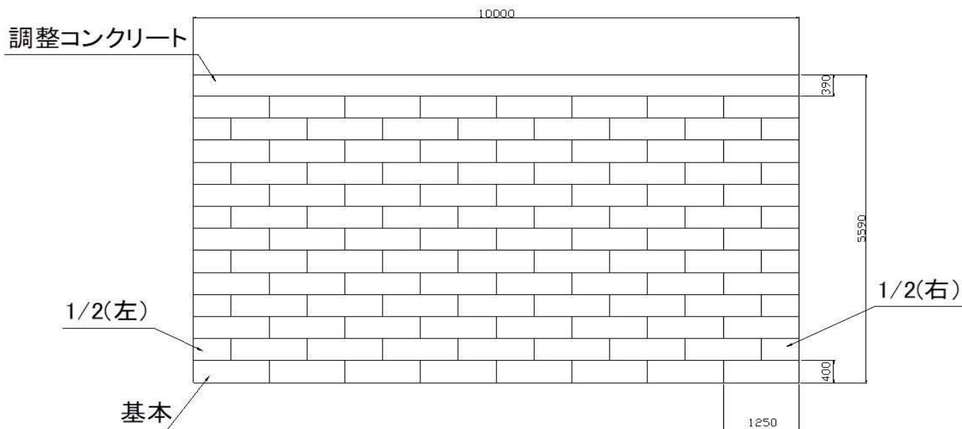
【標準断面図】
