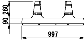
平面図
